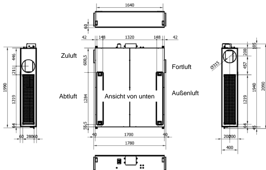
Linke Geräteausführung
