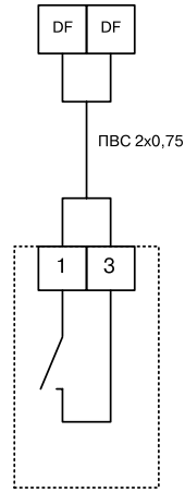
Дифференциальный манометр фильтра
